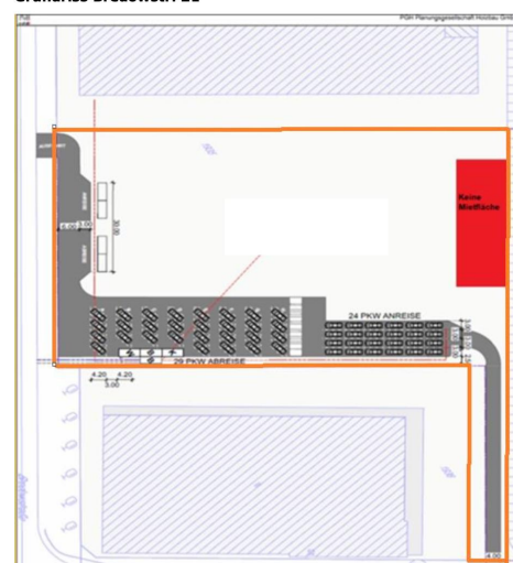
Anlage 1 Grundriss Bredowstr. 21
